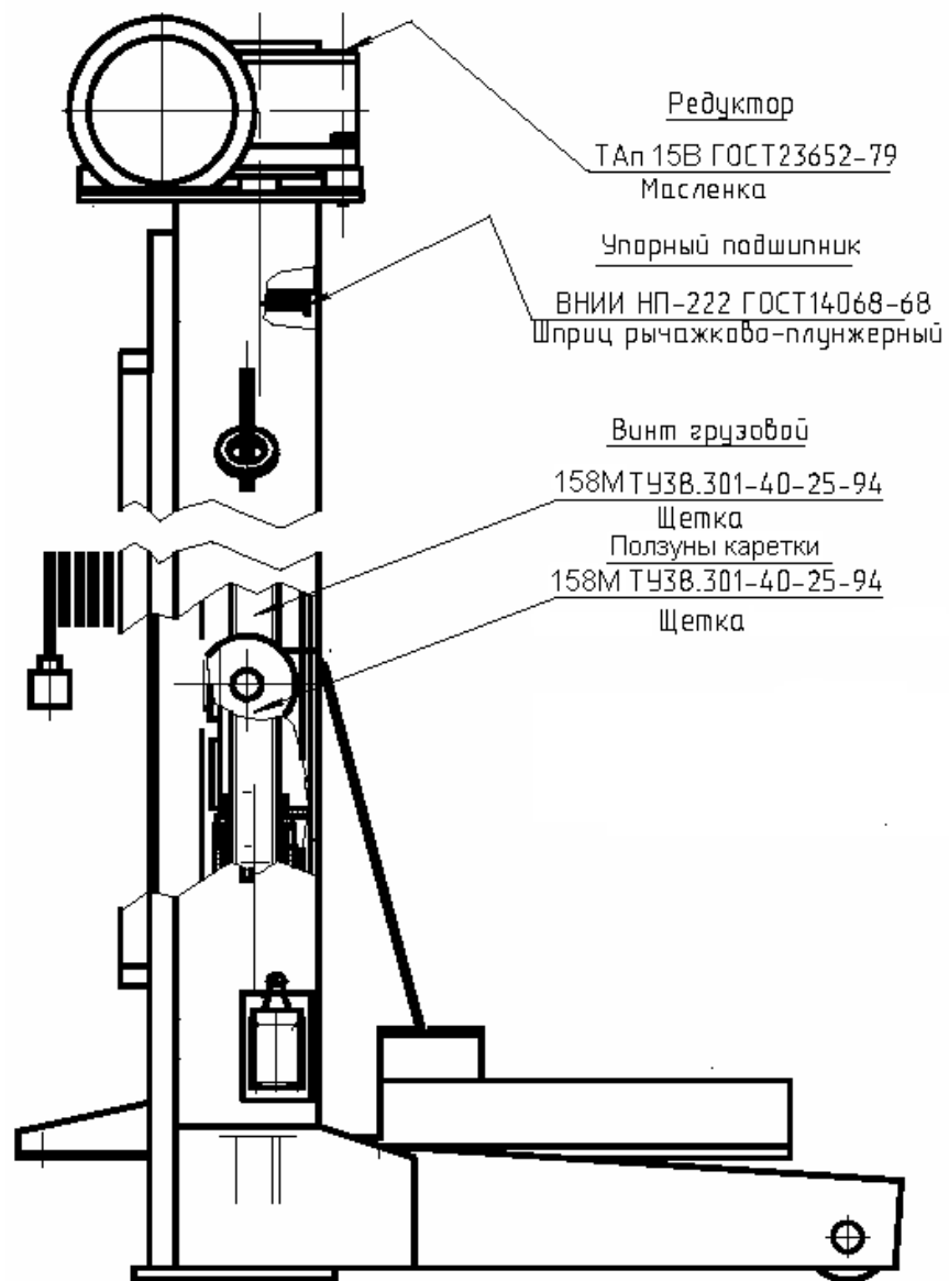
Рис. 6. Карта смазки стойки подъемника ПП-10
